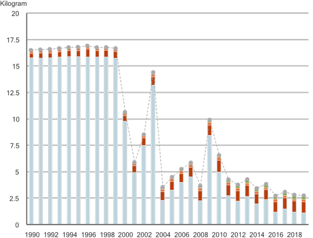
Utsläpp av HCB till luft 1990-2019
