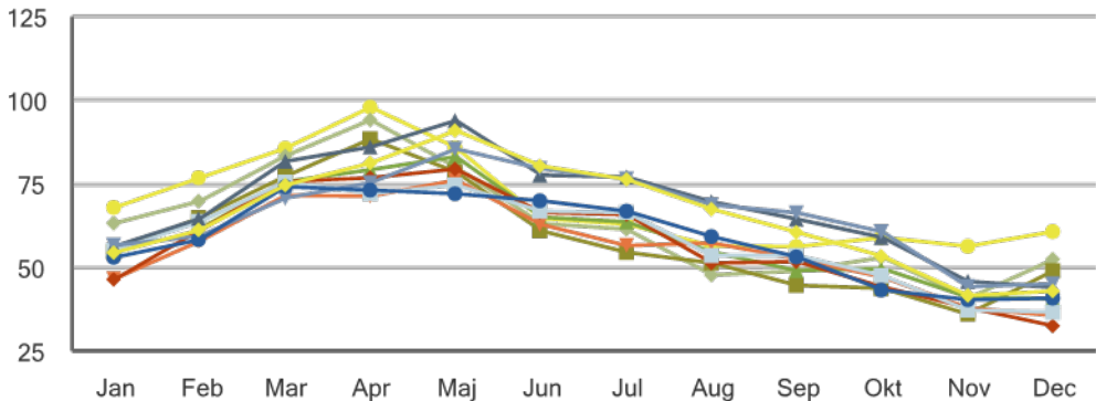
Månadsmedelhalter av ozon i regional bakgrund under 2018
