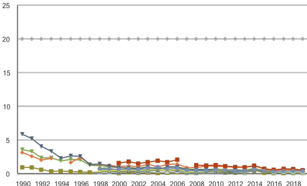
Årsmedelhalter av svaveldioxid i regional bakgrund 1990-2019
