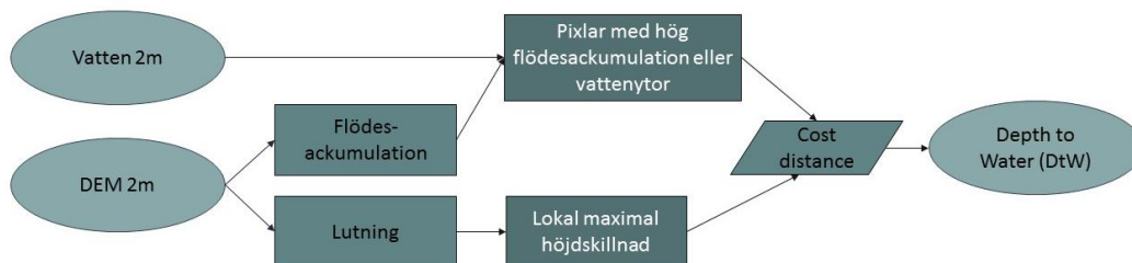
Figur 33. Flödesschema för produktionen av Depth to Water
