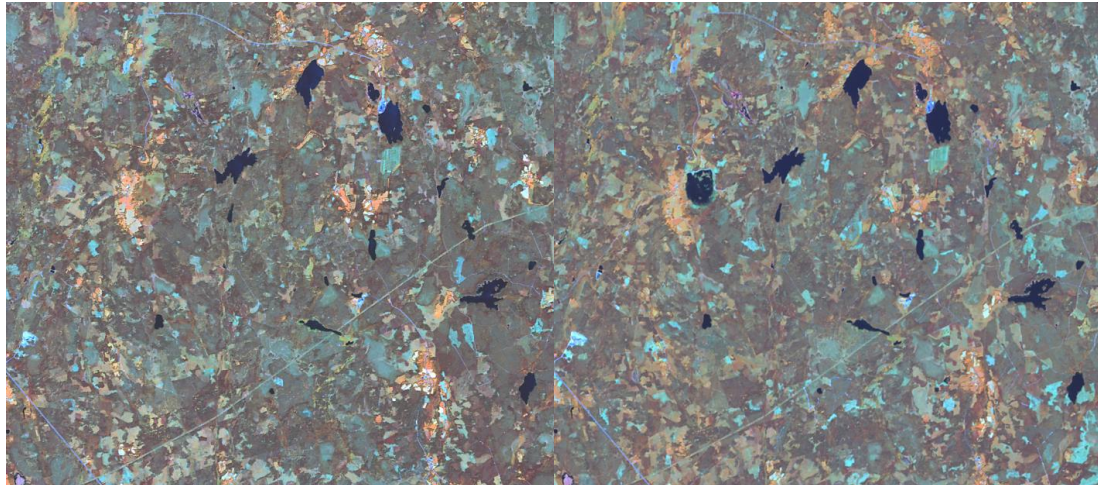
Satellitbildsmosaik SPOT 2010
