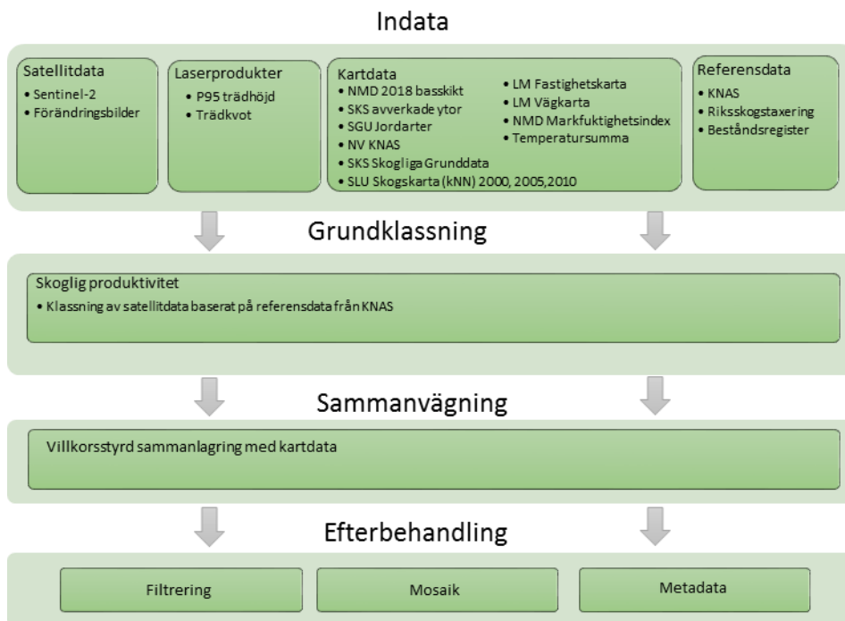
Figur 49. Översiktlig redovisning av produktionsprocessen inom tilläggs-skikt produktivitet.
