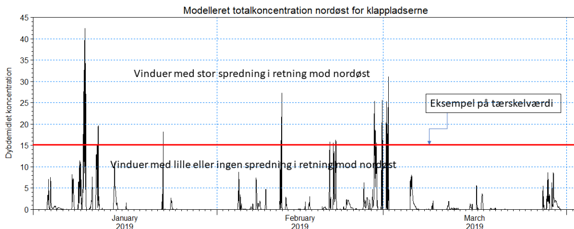
Figur 4 Modelleret tidsserie af den dybdemidlede koncentration (mg/l) i sedimentfanen nordøst for klappladserne.
