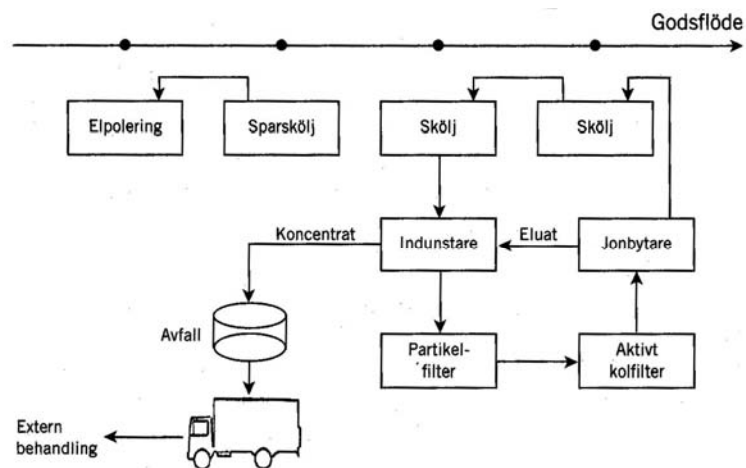
Fig. 39. Avloppsfri elpolering.
