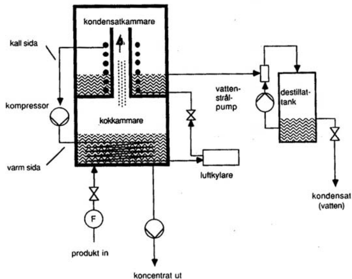
Fig. 29 Vakuumindestare med värmepump för separation av oorganiska salter från vatten.
