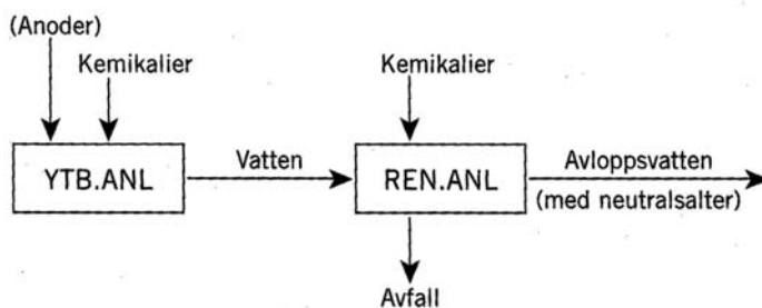
Fig. 25 Vid konventionell end-of-pipe-rening erhålles avloppsvatten innehållande neutralsalter samt ett avfall bestående främst av metallhydroxi-der.
