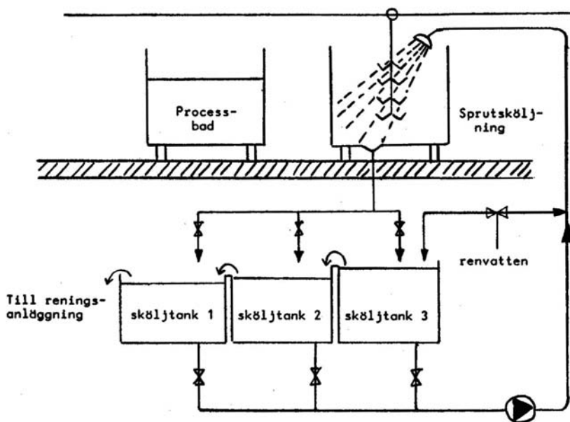
Fig. 4. Motståndssköljning i sköljstation med sköljbaderna placerade i källaren.
