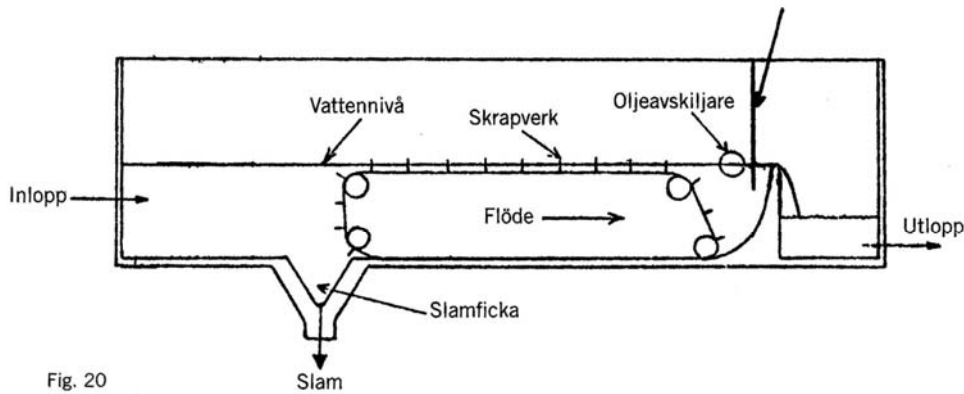
Fig. 20 Exempel på gravitationsavskiljare för fri olja.
