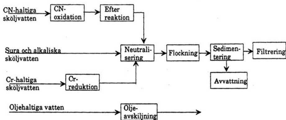
Fig. 6 Exempel på lednings- separation vid renings- anläggning.
