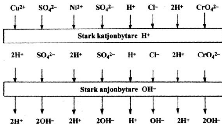
Fig. 28 Vid totalavsaltning byts kat- och anjoner mot väte- respektive hydroxyljoner.
