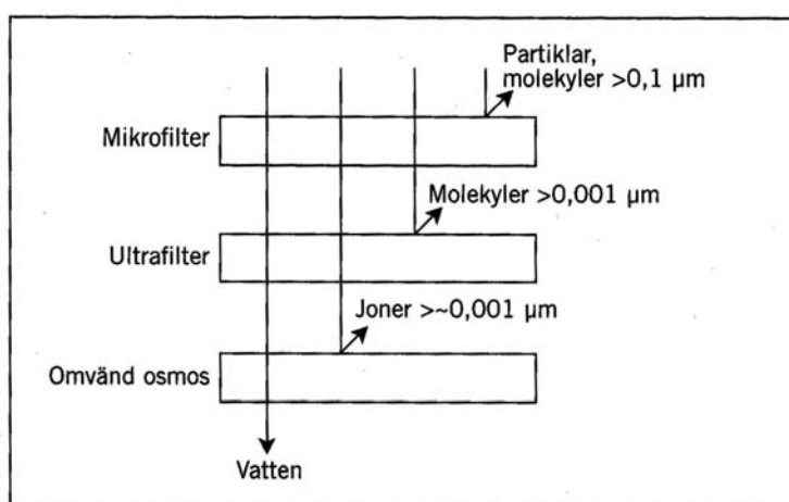
Fig. 31 Avskiljningsområden för några olika typer av membranfiltrering.
