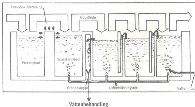
Fig. 3. Trestegs motströmsköljning med sparskölj.
