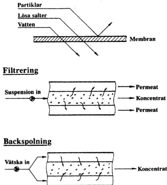
Fig. 24 Mikrofilter, ett alternativ till sandfilter.
