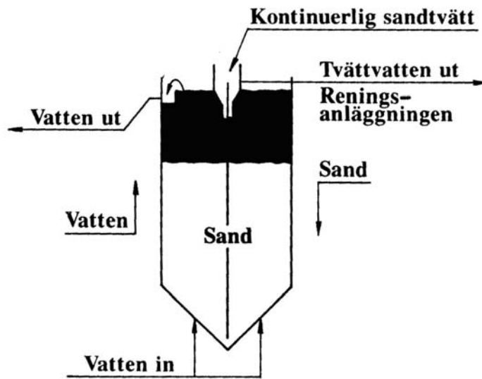
Fig. 23 Kontinuerligt sandfilter.
