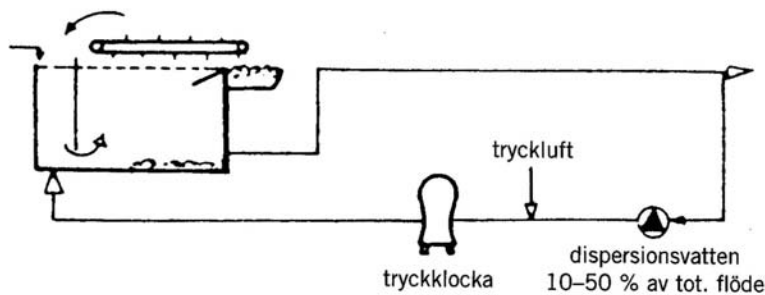
Fig. 14 Flotation, en alternativ avskiljningsmetod.
