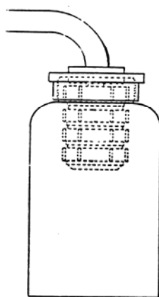
Figur 1 Ett filterpack med tre filter monterade i serie inuti en flaska utan botten. Flaskan fungerar som regnskydd.
